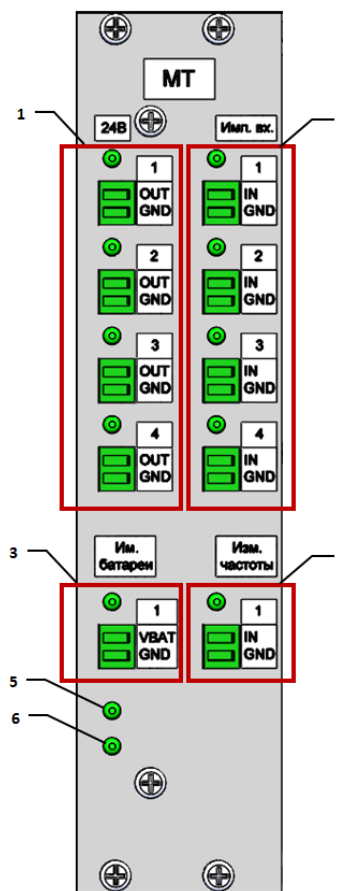
Рисунок 4.8 – лицевая панель МТ
