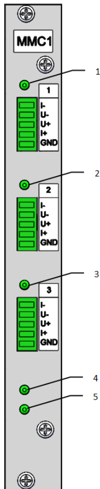
Рисунок 4.2 – Лицевая панель MMC1
